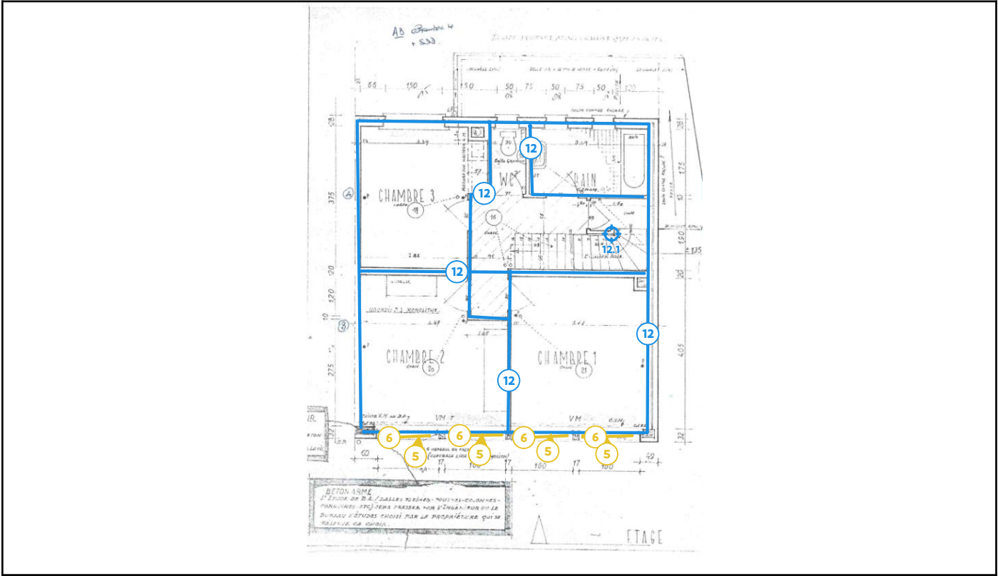
Legende van plan 1.5: Tweede verdieping
